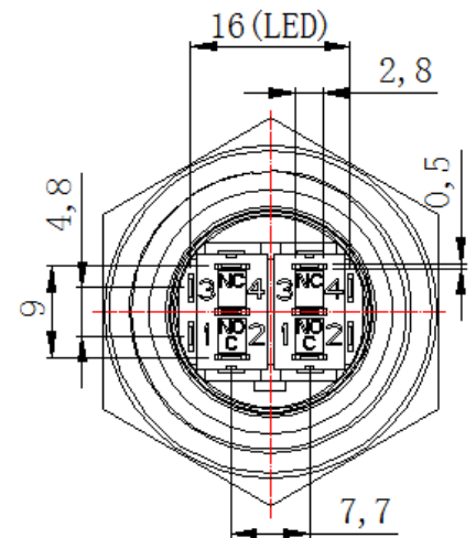
安装孔图
