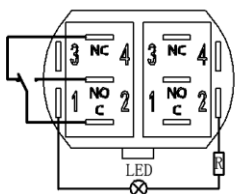
电气简图
