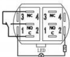
电气简图
