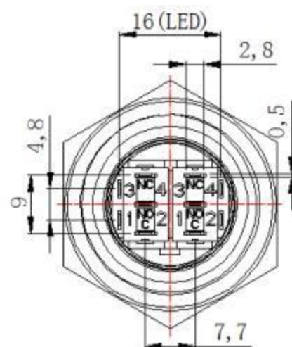
安装孔图
