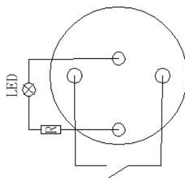
电气简图
