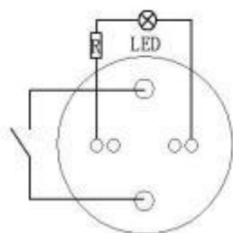
电气简图
