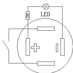
电气简图
