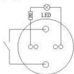
电气简图
