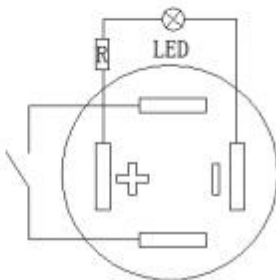
电气简图
