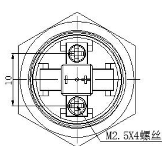
电气简图
