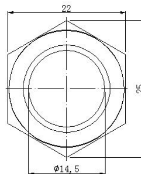
安装孔图
