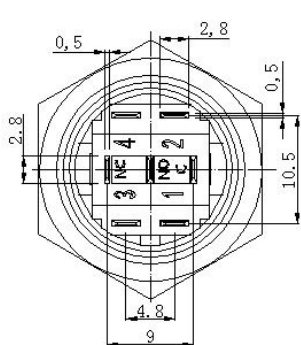
电气简图
