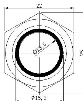
安装孔图
