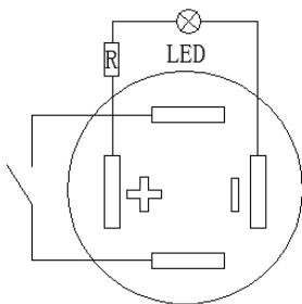
电气简图
